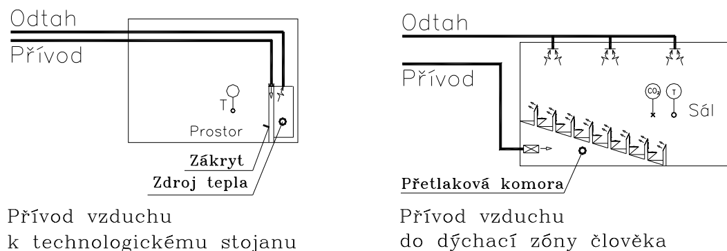
Obr. 4-2: Příklad přívodu vzduchu ke zdrojům škodlivin
