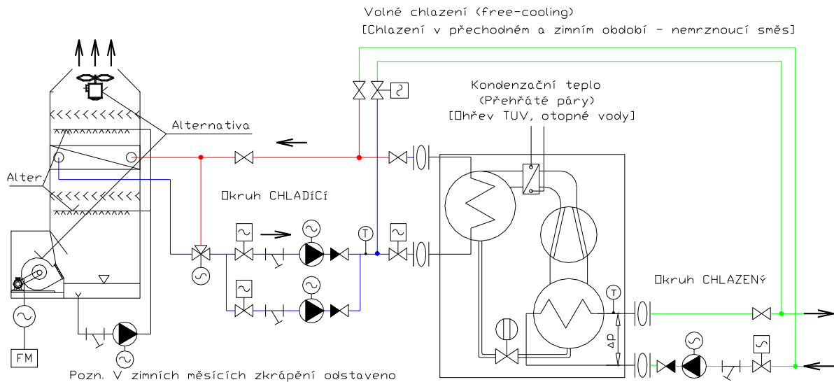
Obr. 3-5: Uzavřená chladicí věž v okruhu strojního chlazení
