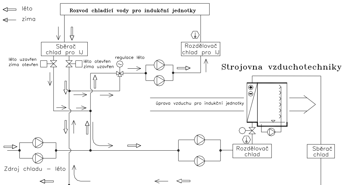
Obr. 3-3: Tepelná smyčka - systém VTK s indukčními jednotkami (IJ)
