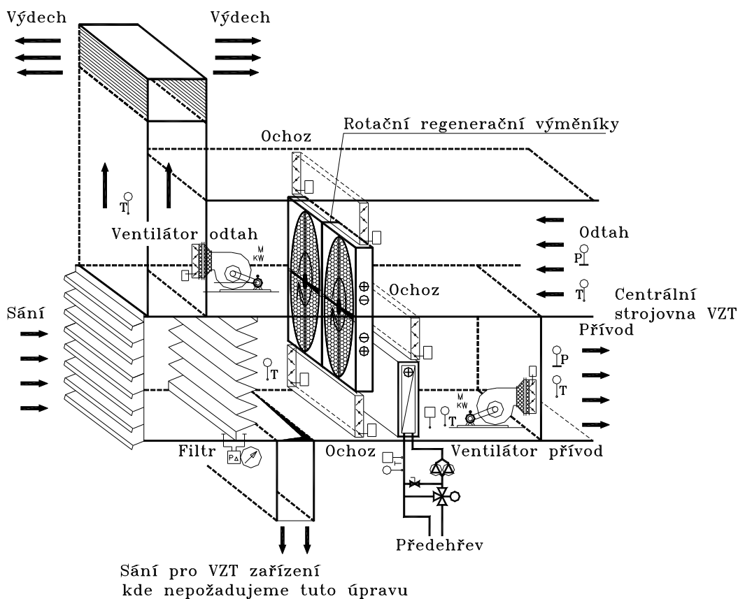
Obr. 3-2: Centrální úprava vzduchu s rotačními regeneračními výměníky.
