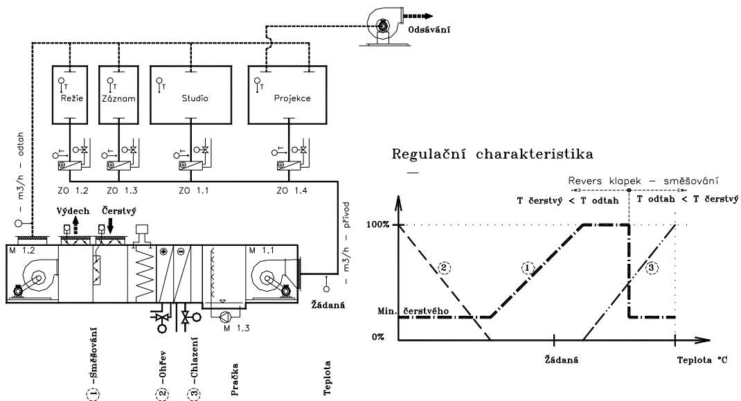
Obr. 3-6: Využití adiabatického chlazení sprchovou pračkou vzduchu pro studiový komplex.
