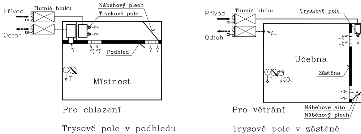
Obr. 4-4: Příklad přívodu vzduchu s proměnlivým množstvím trysovým polem v podhledu nebo zástěně.
