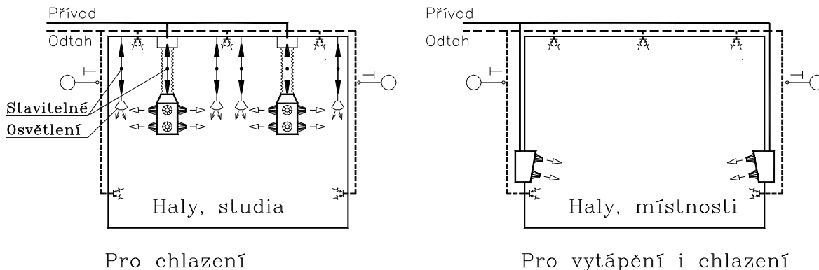
Obr. 4-3: Přívod vzduchu pomocí tryskového pole
