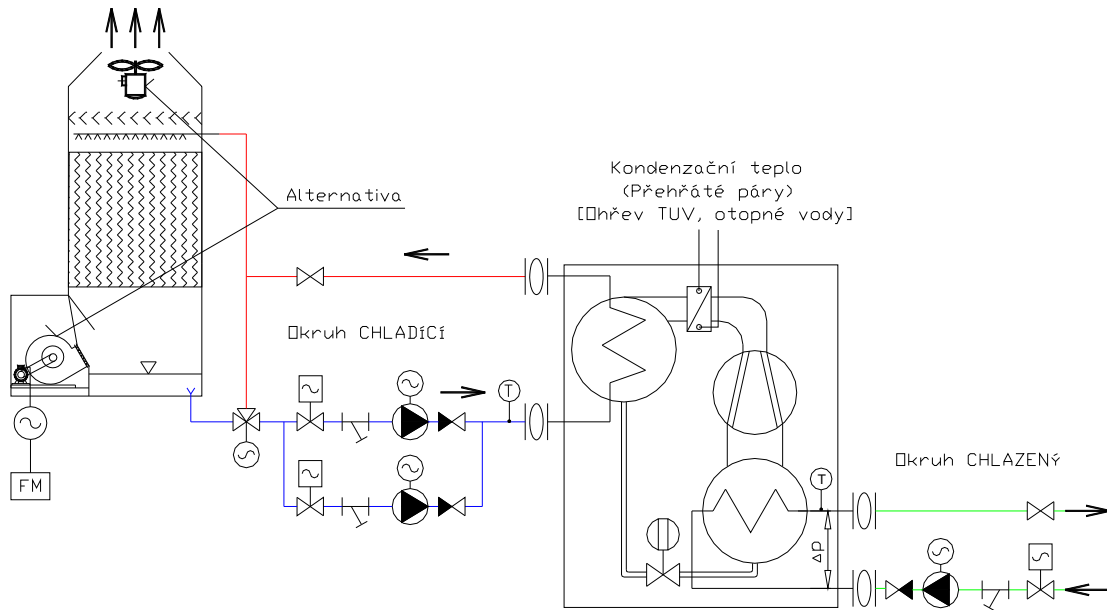
Obr. 3-4: Otevřená chladicí věž v okruhu strojního chlazení
