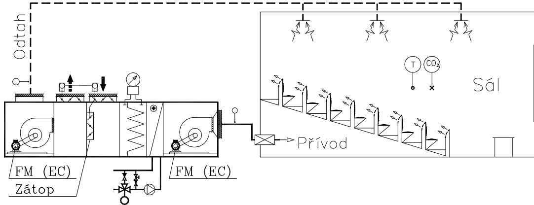
Obr. 4-1: Příklad větrání čerstvým vzduchem s proměnným množstvím vzduchu dle \text{CO}_2 .
