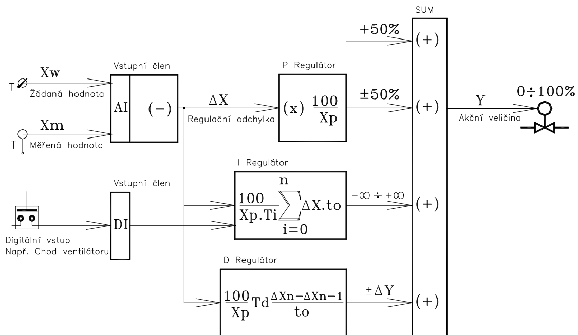
Blokové schéma algoritmu proporcionálně integrační a derivační regulace „PID“
