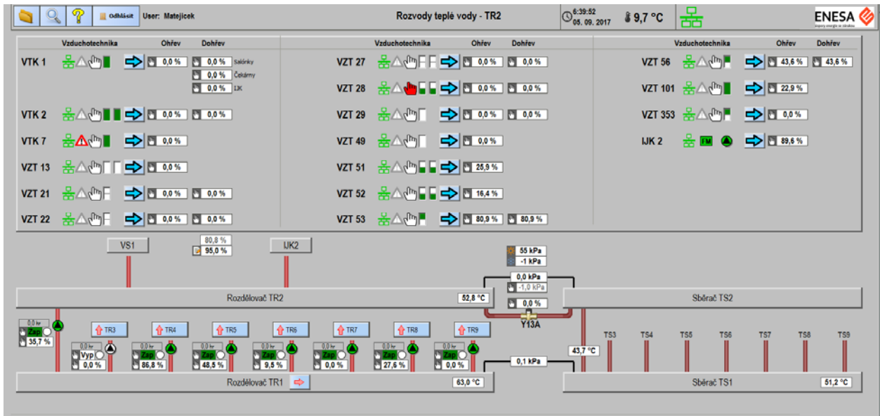
Příklad vizualizace regulace na „Otevřený ventil“
