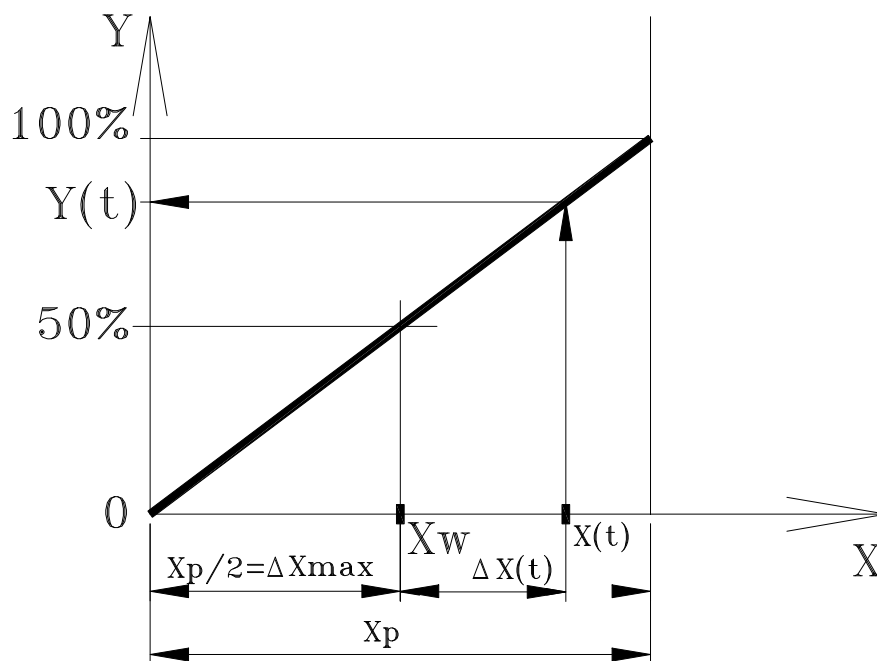
Regulační charakteristika proporcionální regulace - P \Delta X(t) – Trvalá regulační odchylka v čase t , při velikosti akční veličiny Y(t) .
