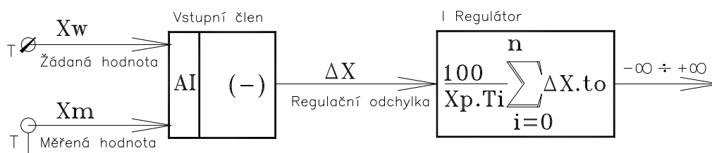
Blokové schéma algoritmu integrační části regulace „I“
