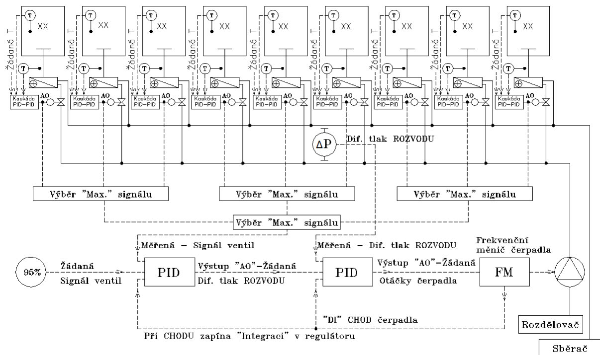
Obr. 11 Regulace otáček na diferenční tlak rozvodných větví teplosměnné látky podle polohy ventilů na „OTEVŘENÝ VENTIL“ z konkrétní aplikace
