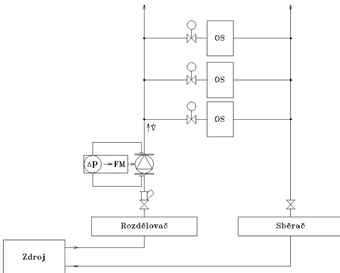
Obr. 3 Řízení otáček oběžného kola čerpadla podle interní tlakové difference
