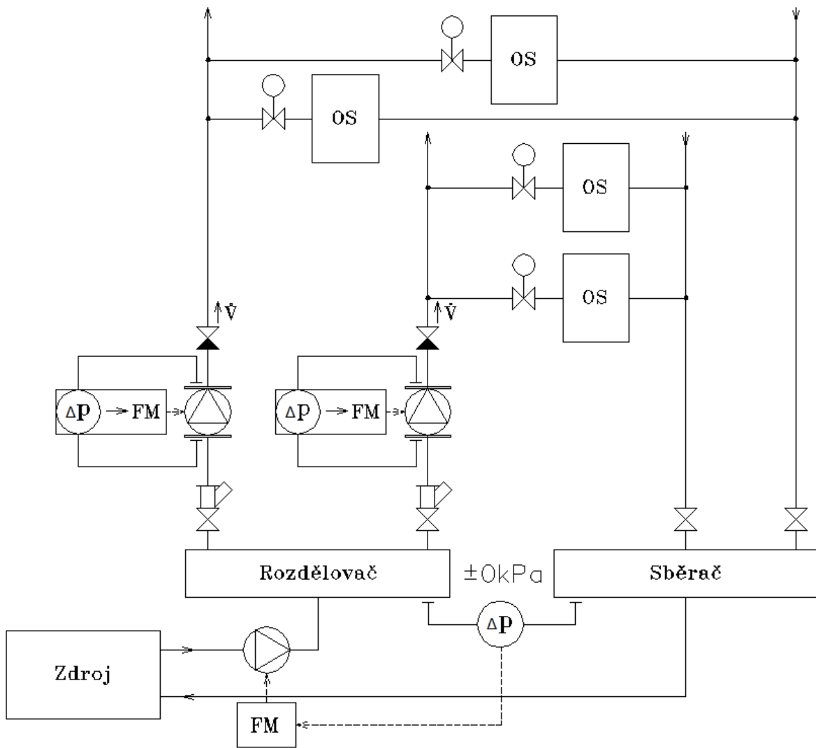
Obr. 6 Řízení otáček čerpadel pro menší soustavy
