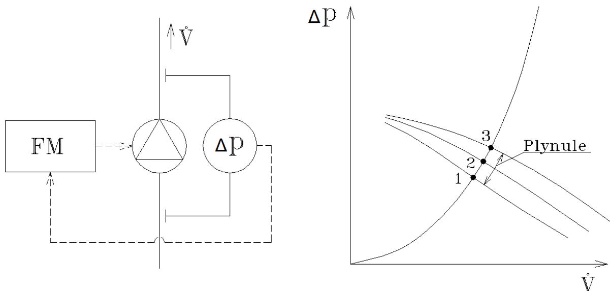
Obr. 1 Čerpadlo s řízením výkonu externím frekvenčním měničem s charakteristikou čerpadla v rozvodné síti teplosměnné látky
