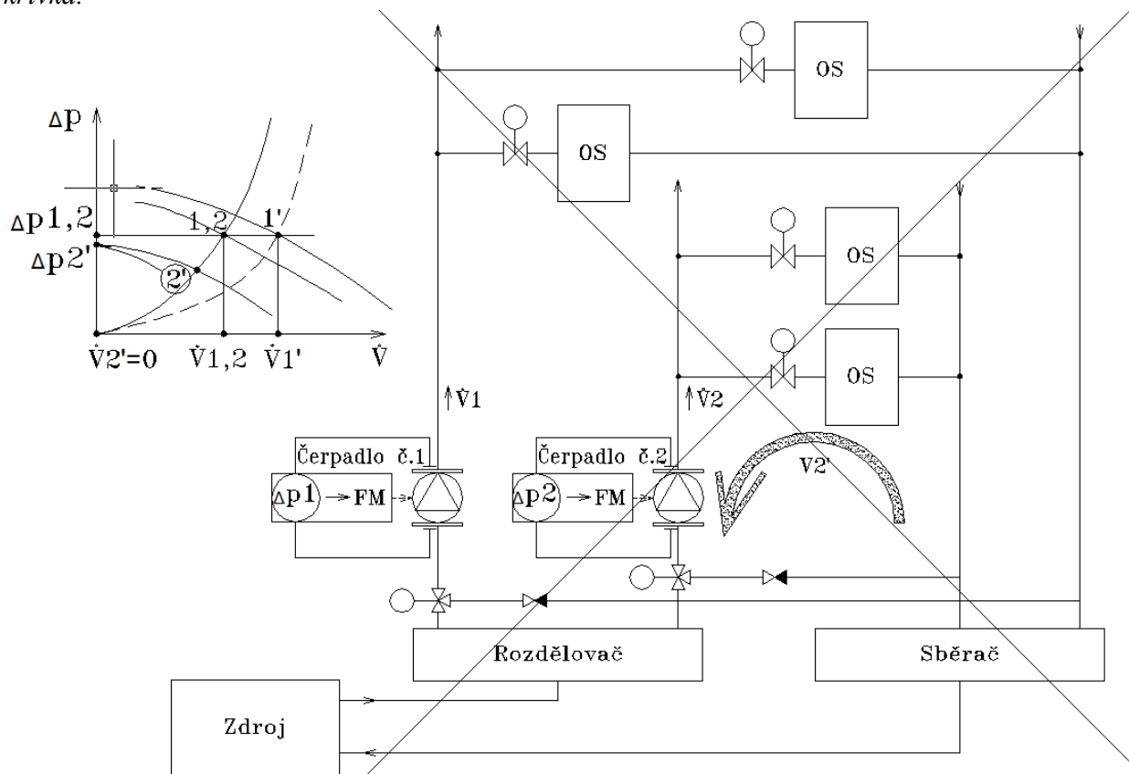
Obr. 4 Řízení otáček oběžného kola čerpadla podle interní tlakové difference pro více, než jeden okruh rozvodu teplosměnné látky
