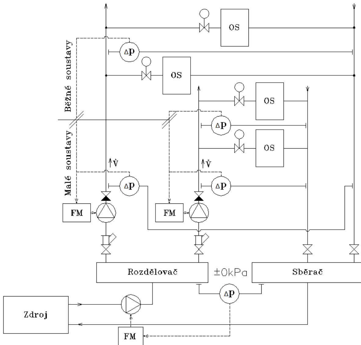
Obr. 7 Řízení otáček čerpadel pro běžné soustavy
