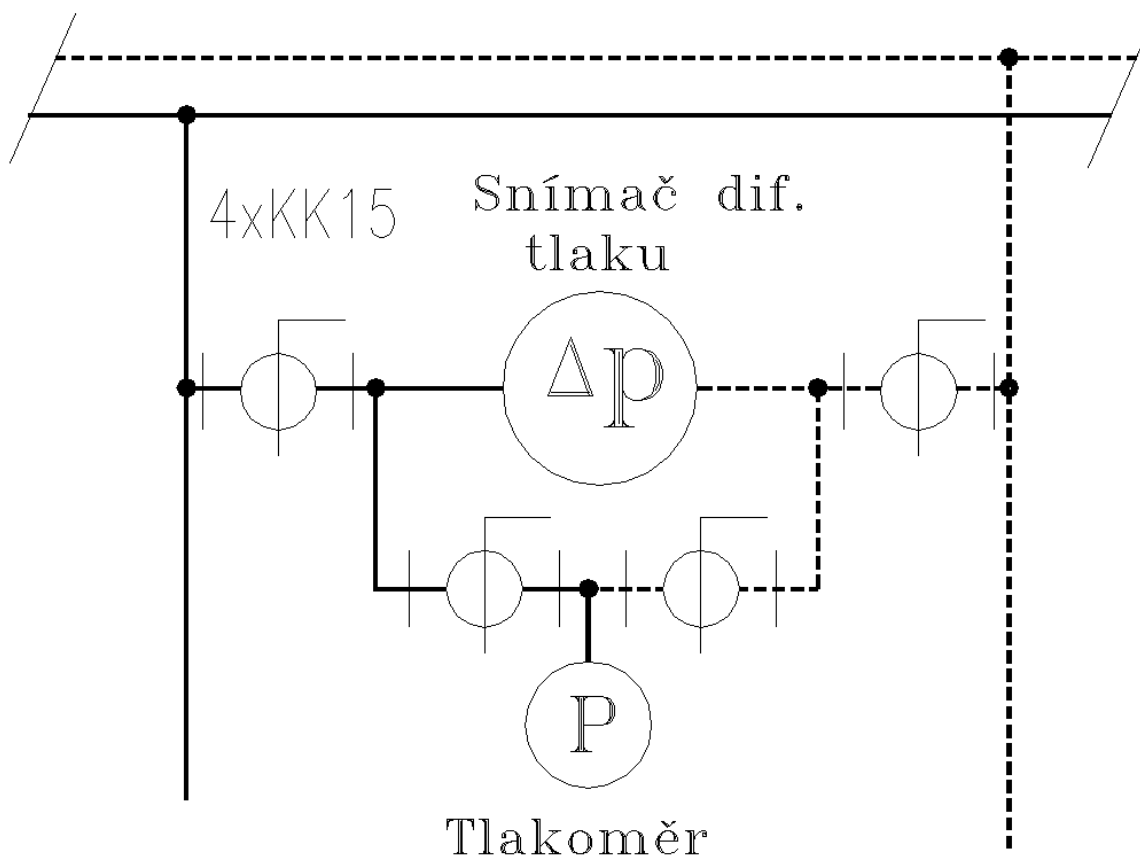
Obr. 12 Příklad zapojení snímače diferenčního tlaku – jednoduchá náhrada šesticečné armatury
