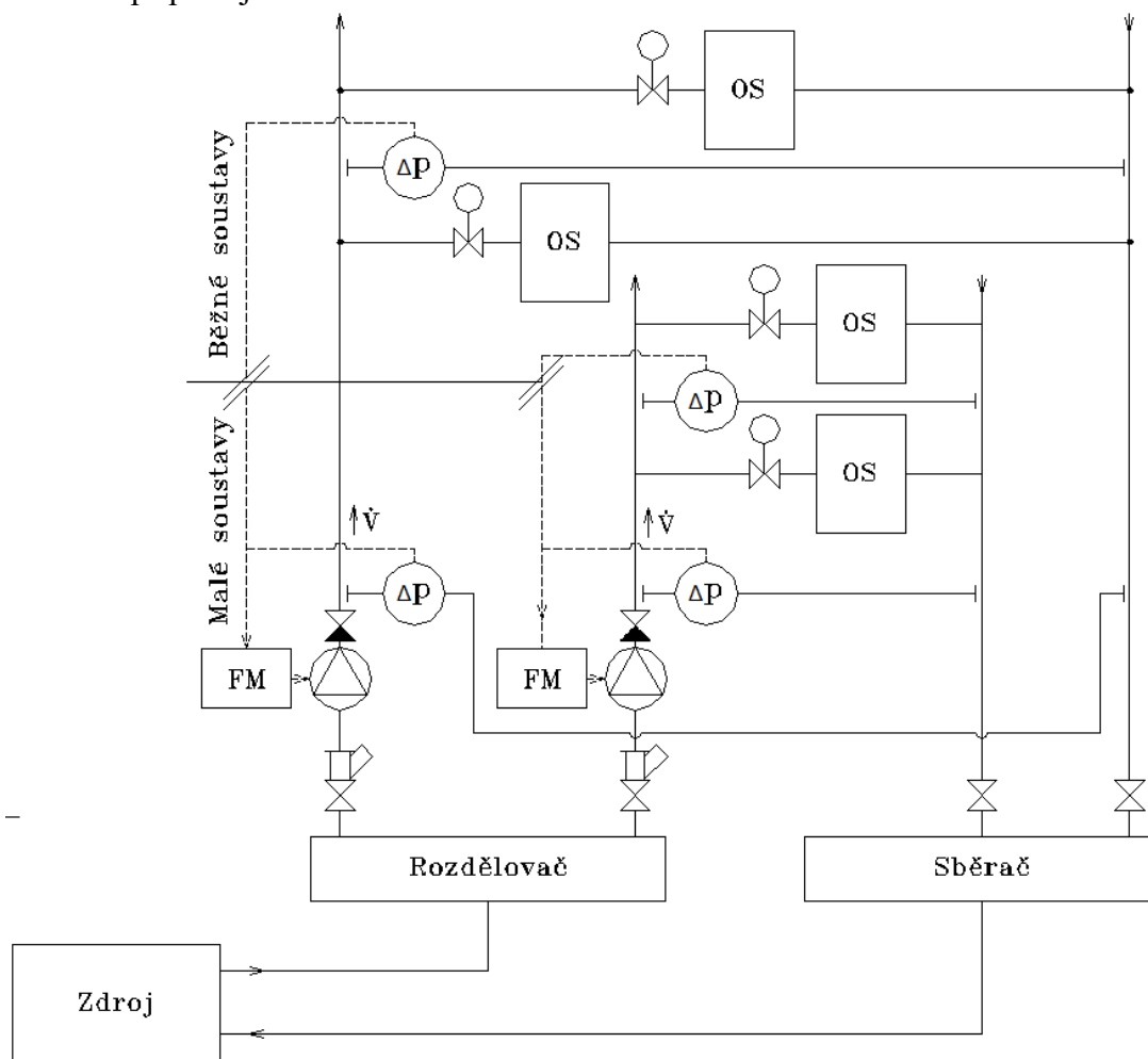
Obr. 5 Řízení otáček oběžného kola čerpadla podle tlakové difference okruhů
