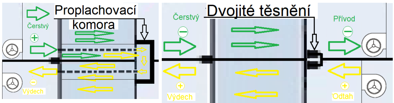
Obr. 3-2.4: Rotační regenerační výměník – požadavek na proplachovací komoru nebo dvojitě těsnění v dělicí rovině kola dle konfiguraci ventilátorů
