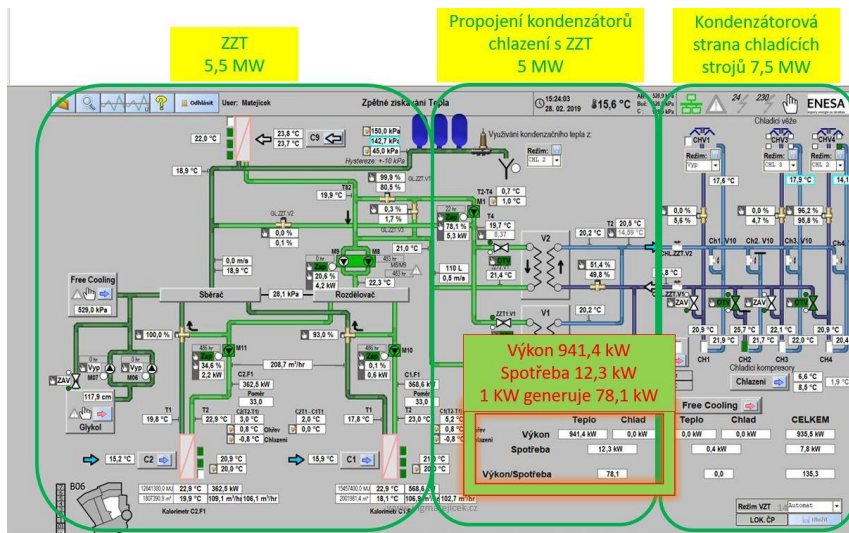
Obr. 3-6: Zpětné získávání tepla kombinované s využitím kondenzačního tepla ze strojního chlazení pro ohřev vzduchu centrální úpravy vzduchu
