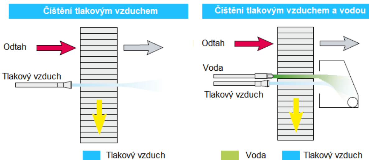
Obr. 3-2.5: Rotační regenerační výměník – údržba, možné čištění kola
