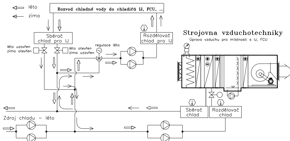
Obr. 3-4: Tepelná smyčka - systém VTK s indukčními jednotkami (IJ), FCU
