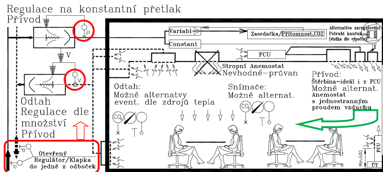
Obr. 5.1 Ideální distribuce vzduchu ve velkoplošných kancelářích
