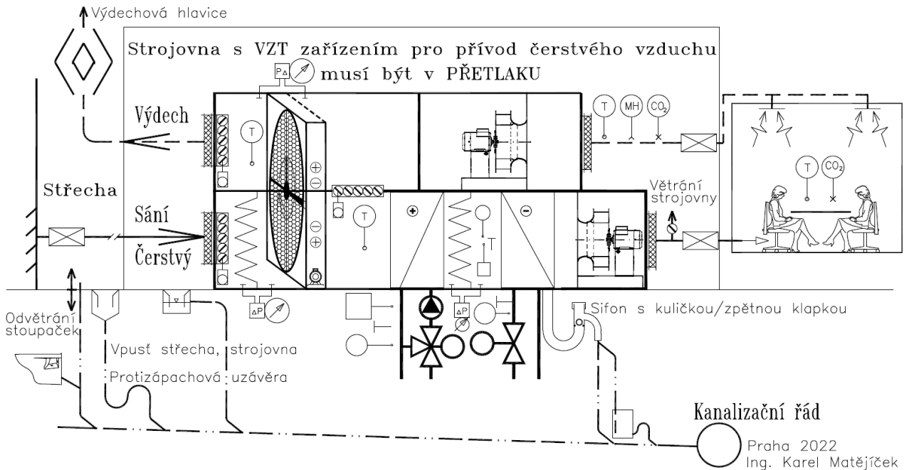
Obr.: 6.2 Vzduchotechnická jednotka versus kanalizace
