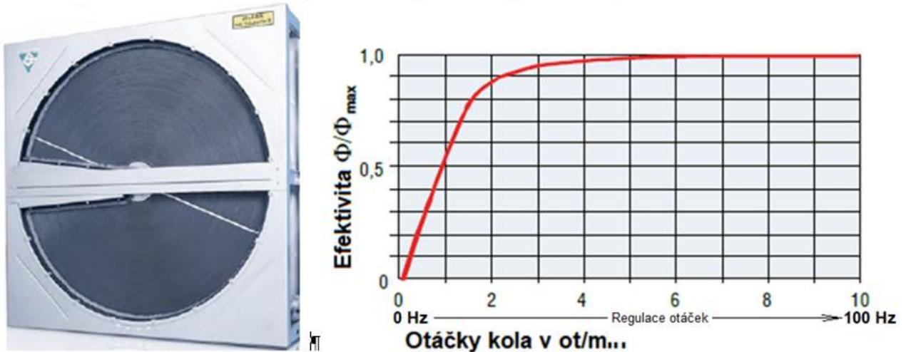
Obr. 3-2.1: Rotační regenerační výměník – závislost efektivity přenosu na otáčkách kola
