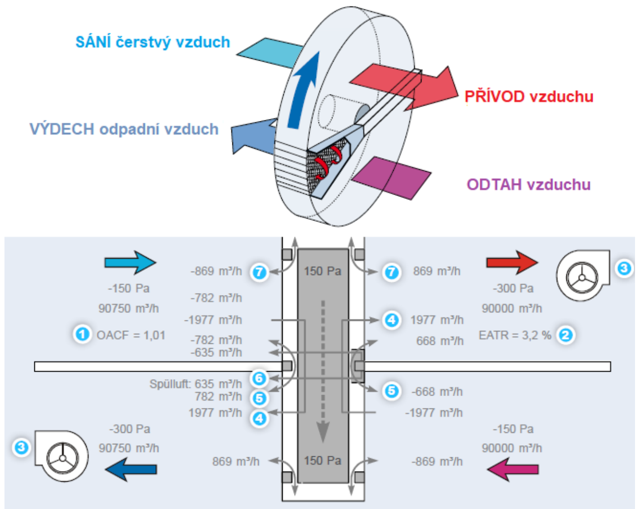
Obr. 3-2.2: Rotační regenerační výměník – příklad naměřených množství vzduchu pronikajících netěsnostmi v konfiguraci ventilátor přívod za kolem a odtah také za kolem – vždy ve směru proudu vzduchu
