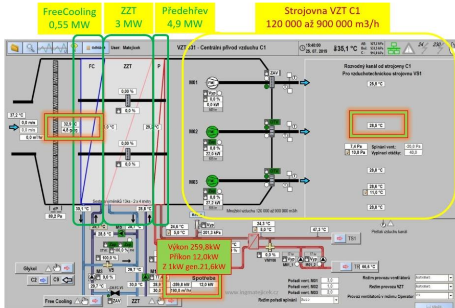
Obr. 3-5: Instalace výměníků pro centrální úpravu vzduchu pro Free Cooling, ZZZ a přehřev
