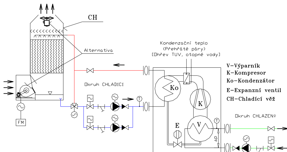
Obr. 3-9: Otevřená chladicí věž v okruhu strojního chlazení
