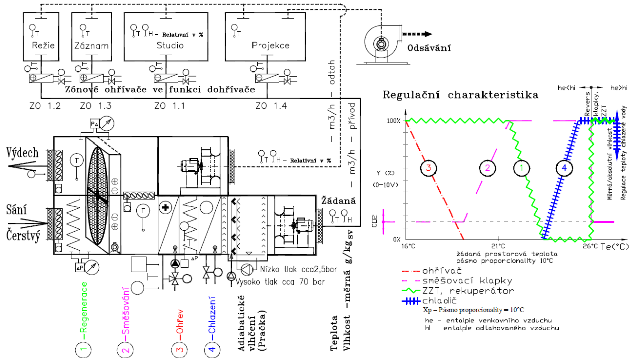
Obr. 3-8: Využití adiabatického chlazení sprchovou pračkou vzduchu pro studiový komplex.
