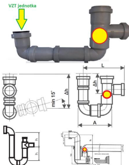
Obr.: 6.3 Příklad sifonu pro připojení odvodů kondenzátu VZT zařízení do kanalizace
