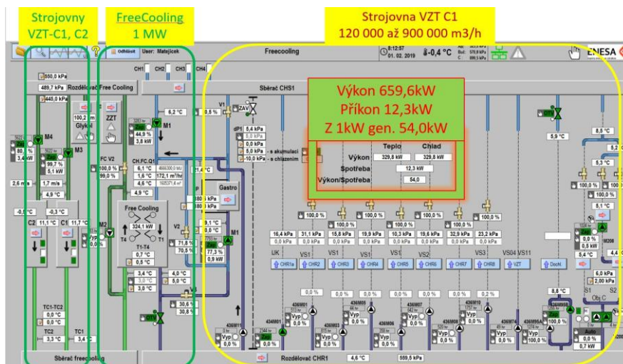
Obr. 3-7: Výroba chladu systémem Free Cooling s využitím tepla pro ohřev vzduchu centrální úpravy vzduchu
