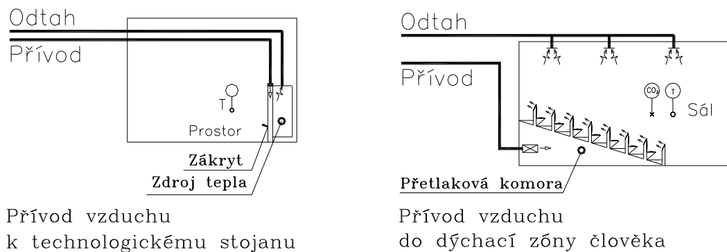
Obr. 4-2: Příklad přívodu / odtahu vzduchu ke / od zdrojům škodlivin
