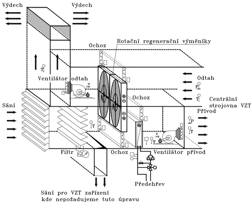
Obr. 3-3: Centrální úprava vzduchu s rotačními regeneračními výměníky.
