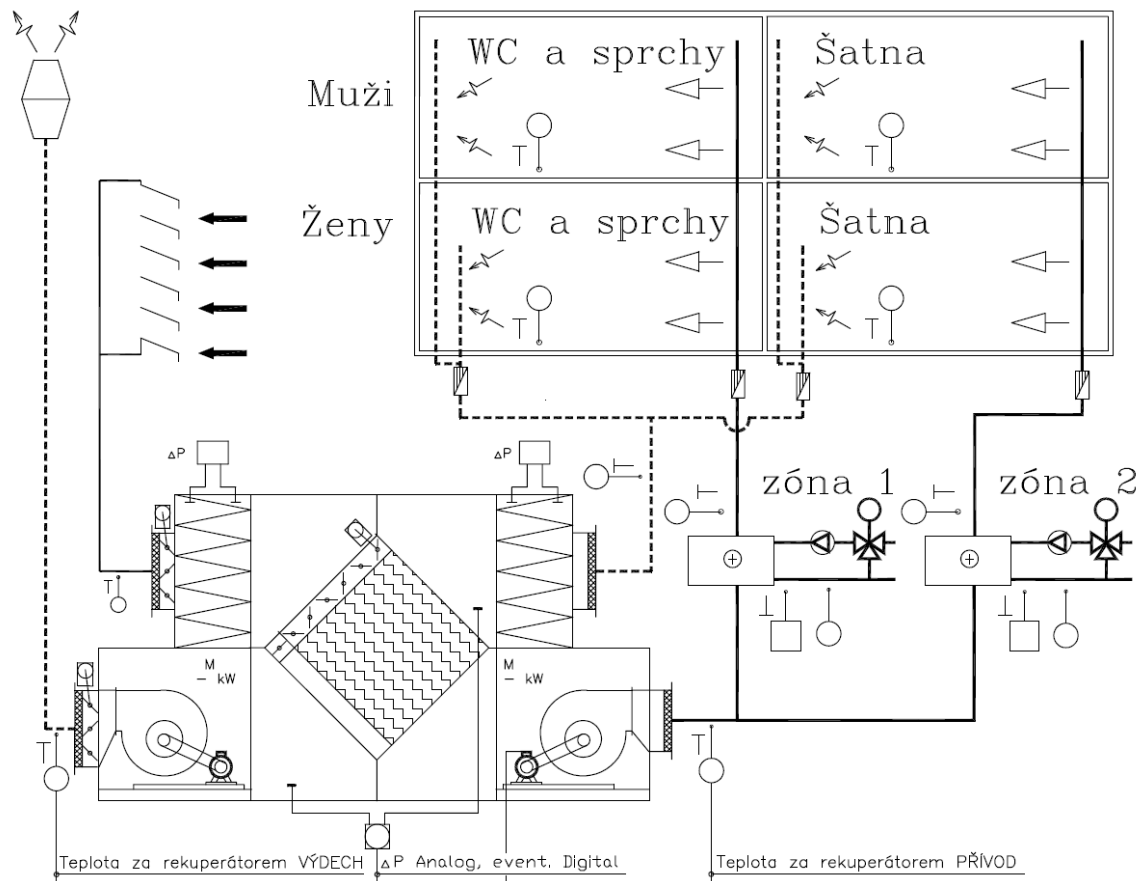
Příklad regulace křížového výměníku vzduch – vzduch
