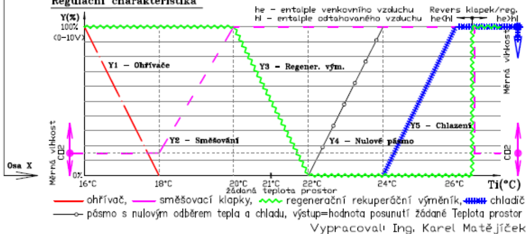
Regulační charakteristika
