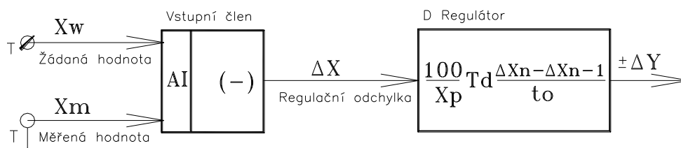
Blokové schéma algoritmu derivační regulace „D“
