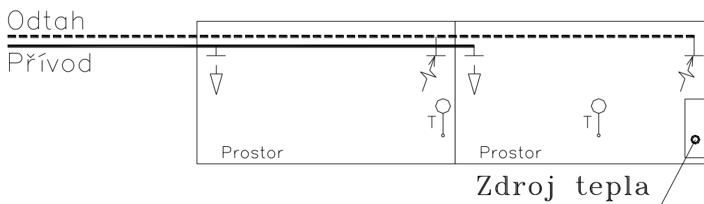
Vhodné umístění čidla v prostoru
