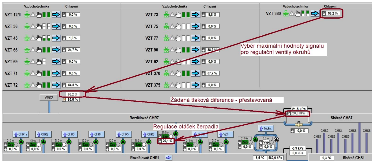
Příklad vizualizace regulace na „Otevřený ventil“
