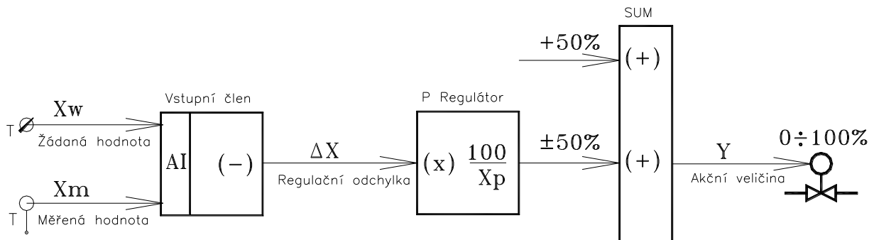
Blokové schéma algoritmu proporcionální regulace „P“
