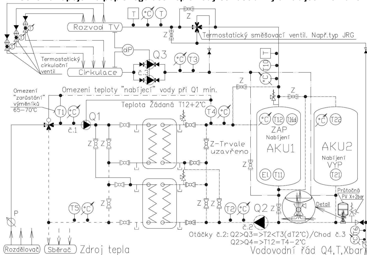
Schéma zapojení a popis regulace Teplé vody se zásobníky a nabíjecím okruhem
