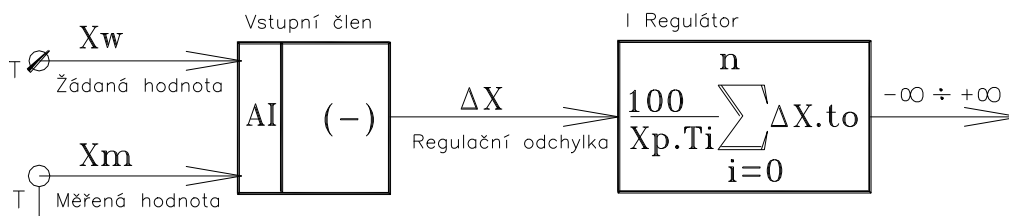
Blokové schéma algoritmu integrační části regulace „I“
