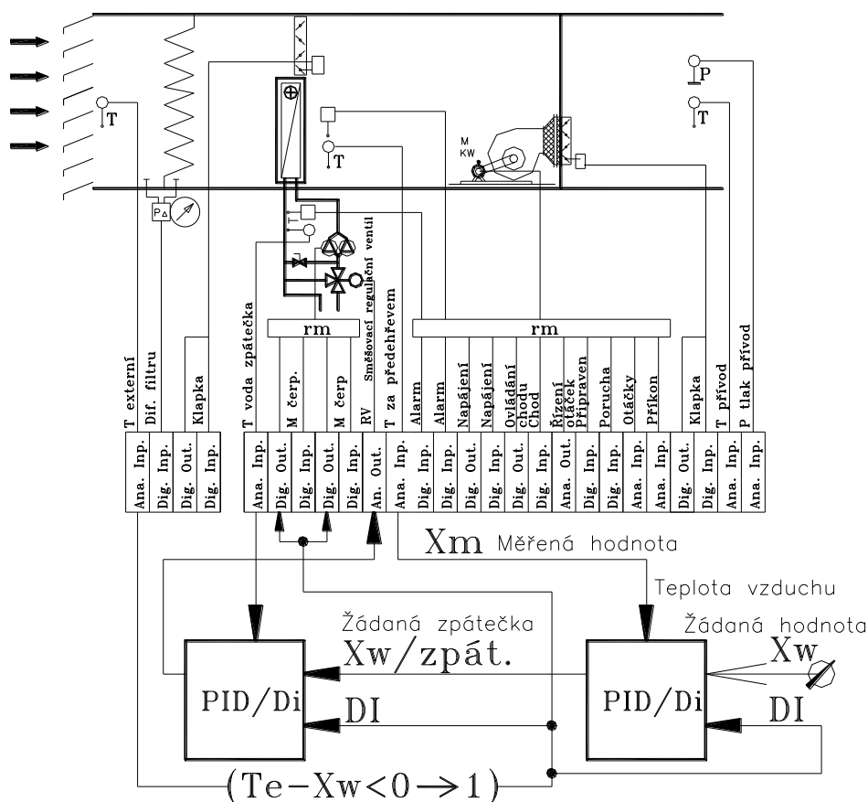
Schéma centrální úpravy vzduchu bez rekuperace s regulací kaskáda PID, PID.
