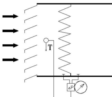
VZT zařízení pro filtraci vzduchu
