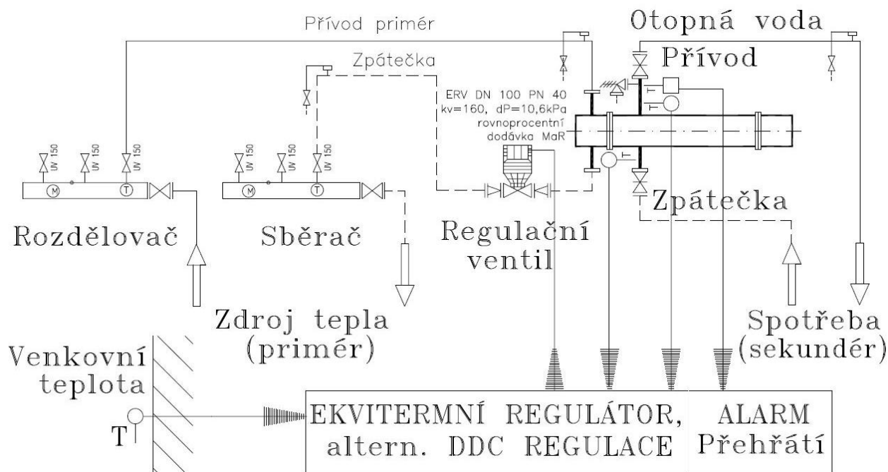
Schéma regulace ÚT VM stanice
