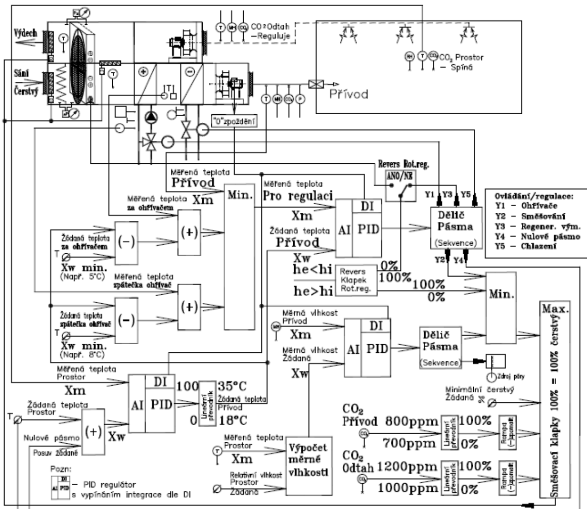
Regulační charakteristika
