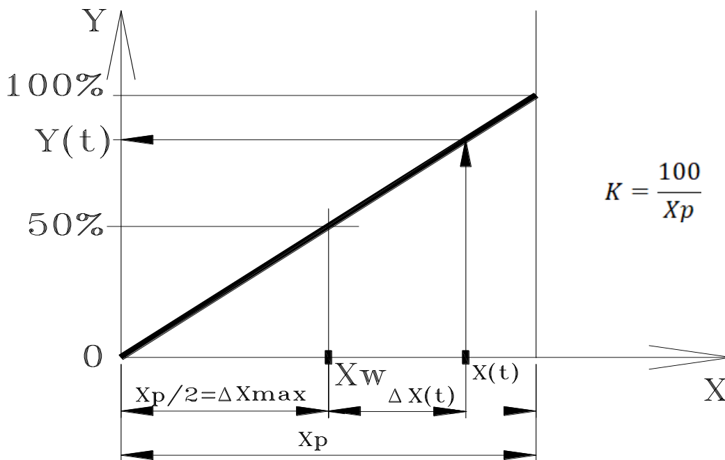
Regulační charakteristika proporcionální regulace - P
