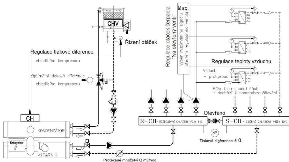
Obr. 4 Rozvody chlazené vody s dvojcestnými regulačními ventily u spotřeby a propojovací potrubí mezi rozdělovačem a sběračem
