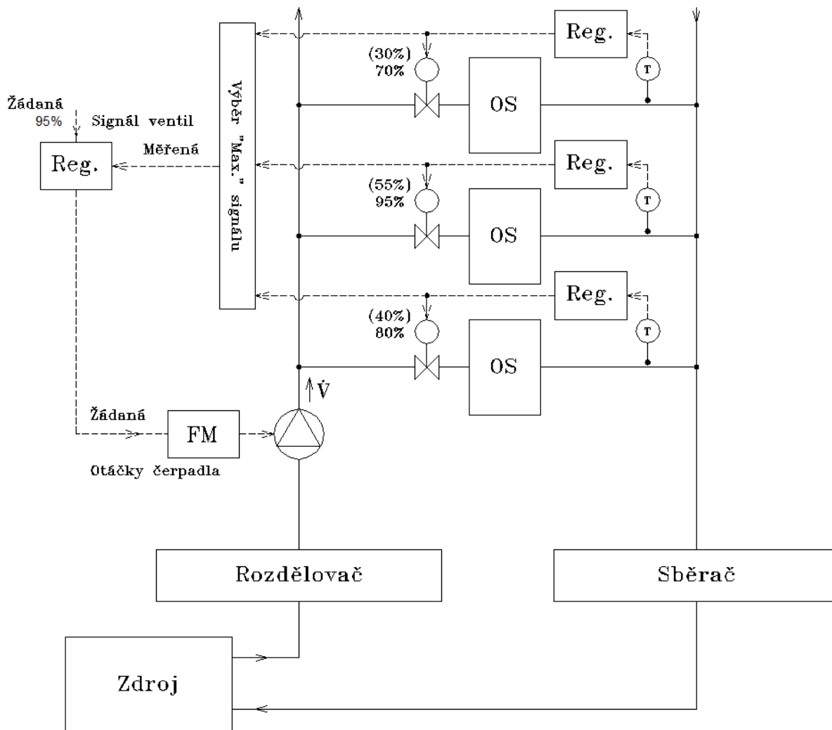
Obr. 2 Regulace otáček na „OTEVŘENÝ VENTIL“
