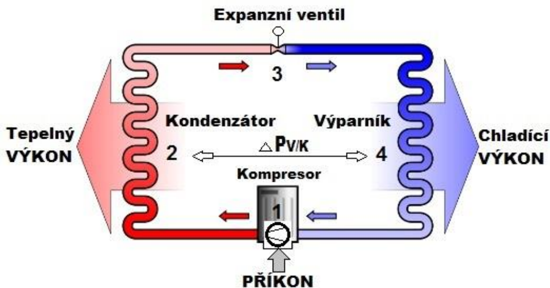
Obr. 1 Okruh kompresorového chladicího stroje
