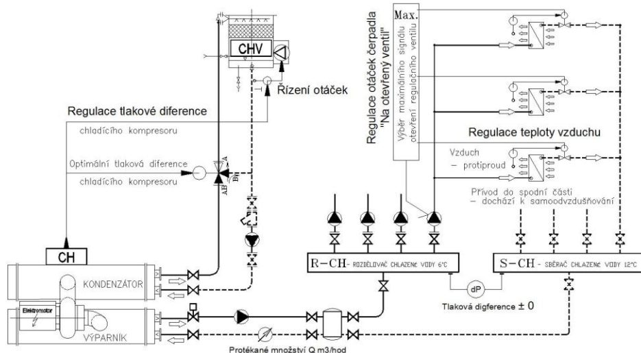
Obr. 5 Rozvody chlazené vody s dvojcestnými regulačními ventily u spotřeby a termohydraulickým rozdělovačem – nejméně vhodná varianta
