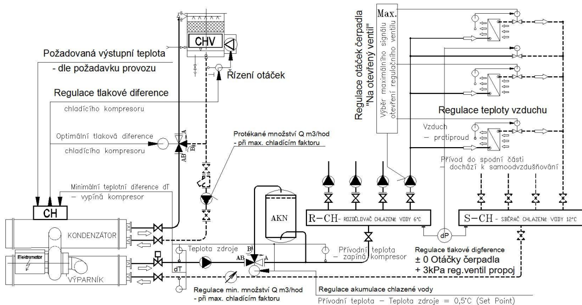
Obr. 8 Rozvody chlazené vody s dvojcestnými regulačními ventily, regulovaným přepouštěním na koncích větví a akumulační nádrží v přívodní větvi
