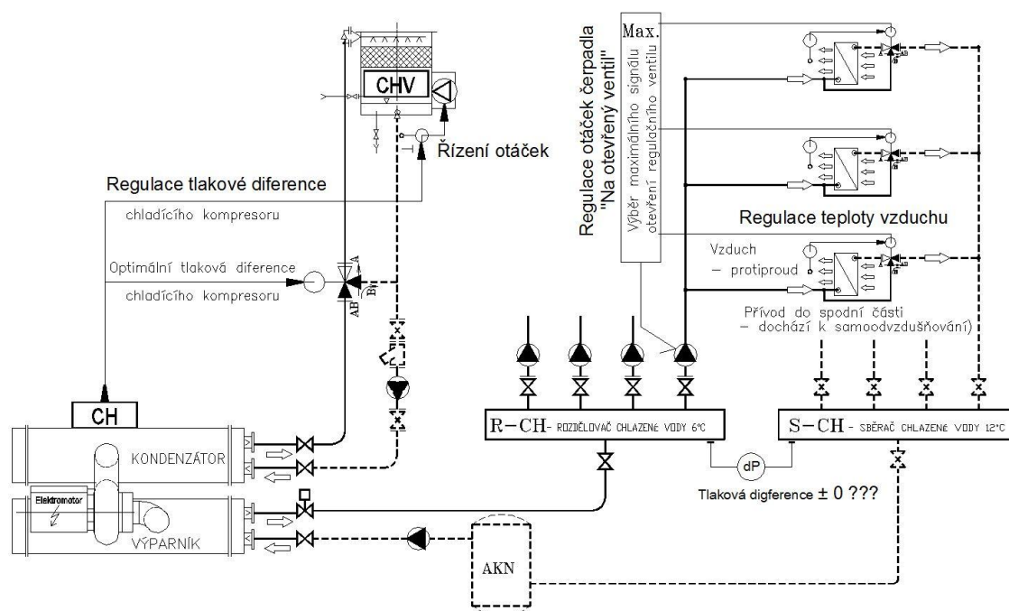
Obr. 6 Rozvody chlazené vody s trojcestnými regulačními ventily u spotřeby a akumulární nádrží ve zpátečce
