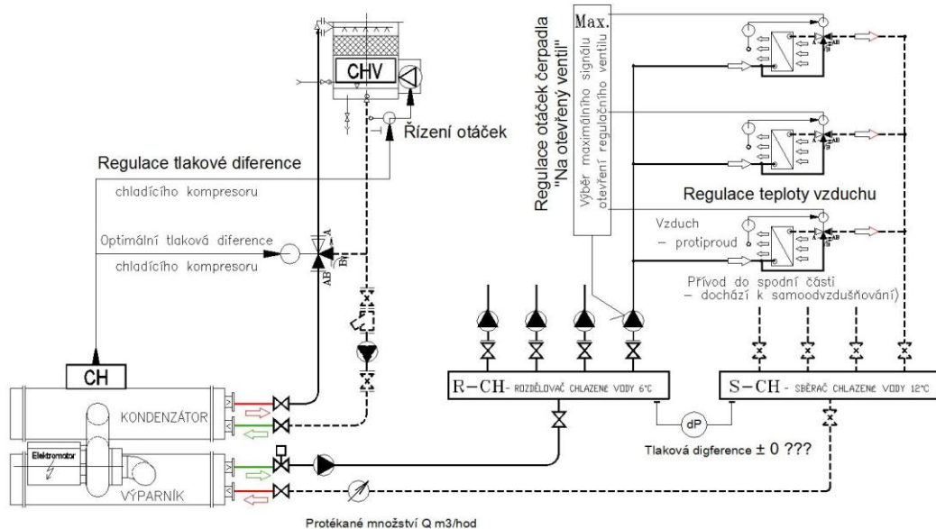
Obr. 3 Rozvody chlazené vody s trojcestnými regulačními ventily u spotřeby
